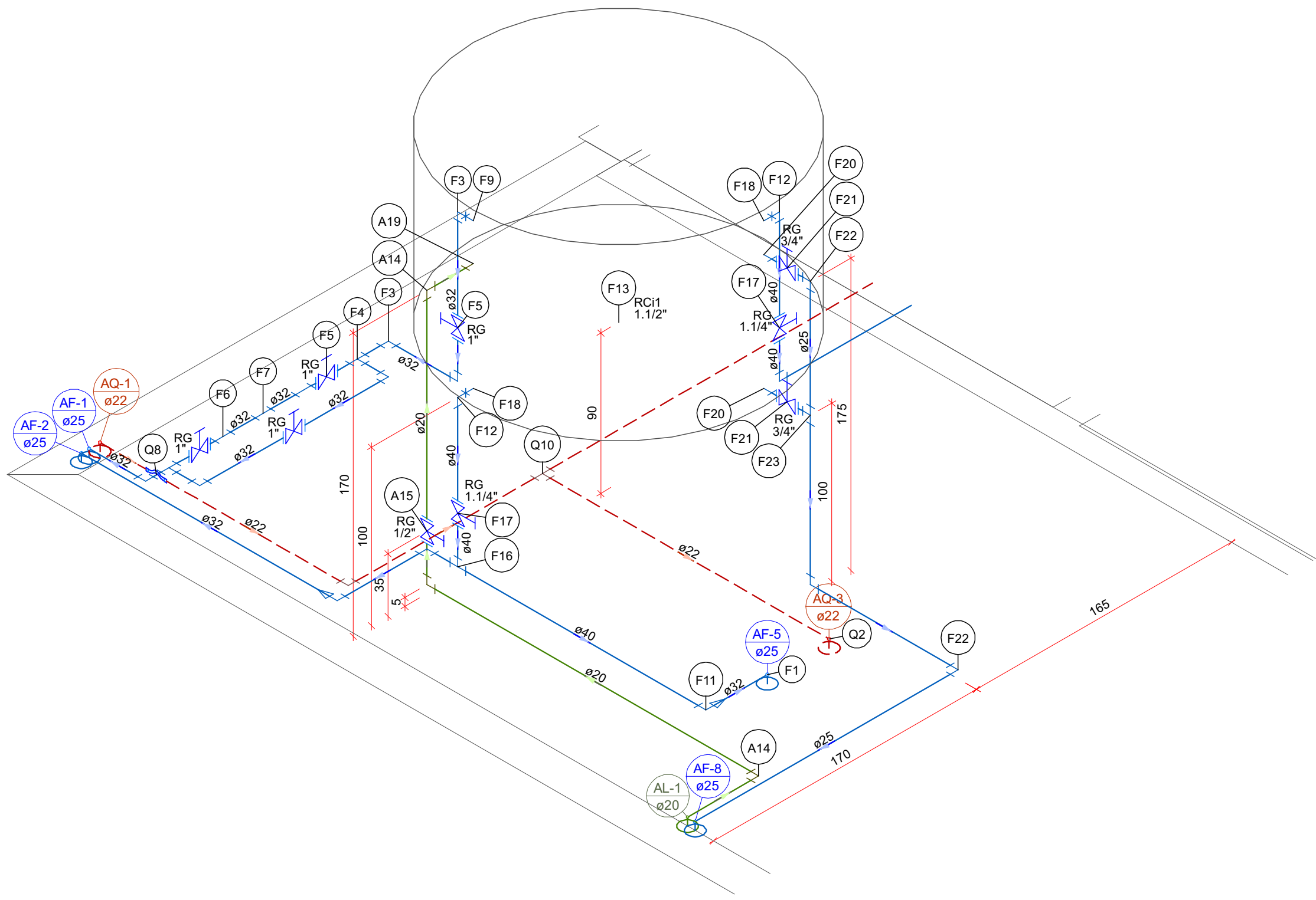
Detalhe Hidráulico-14 Escala 1:25
