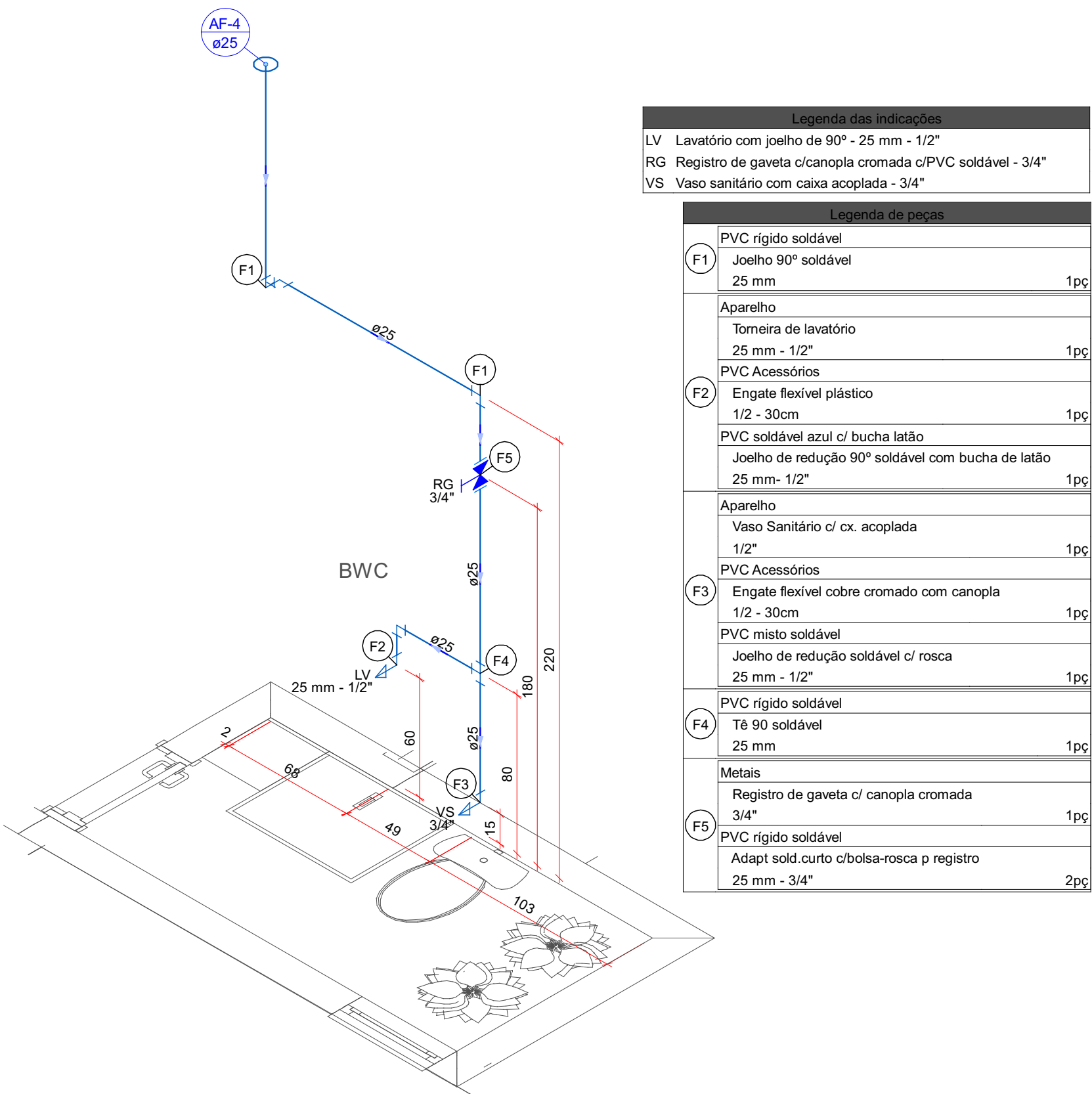
Detalhe Hidráulico-5 Escala 1:25
