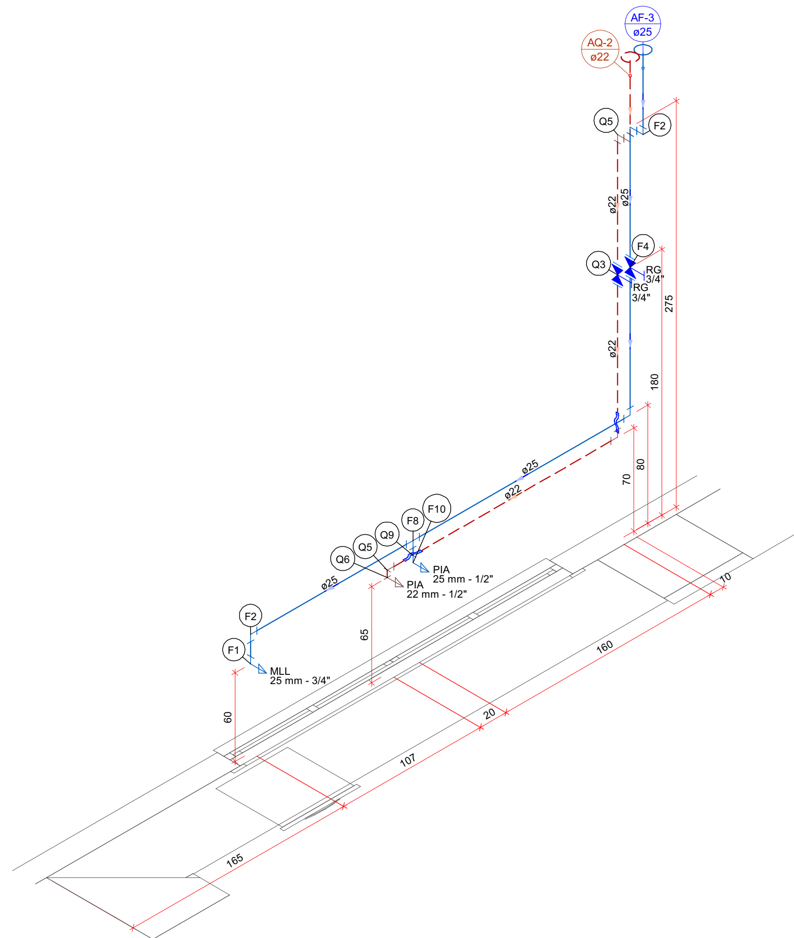
Detalhe Hidráulico-2 Escala 1:25
