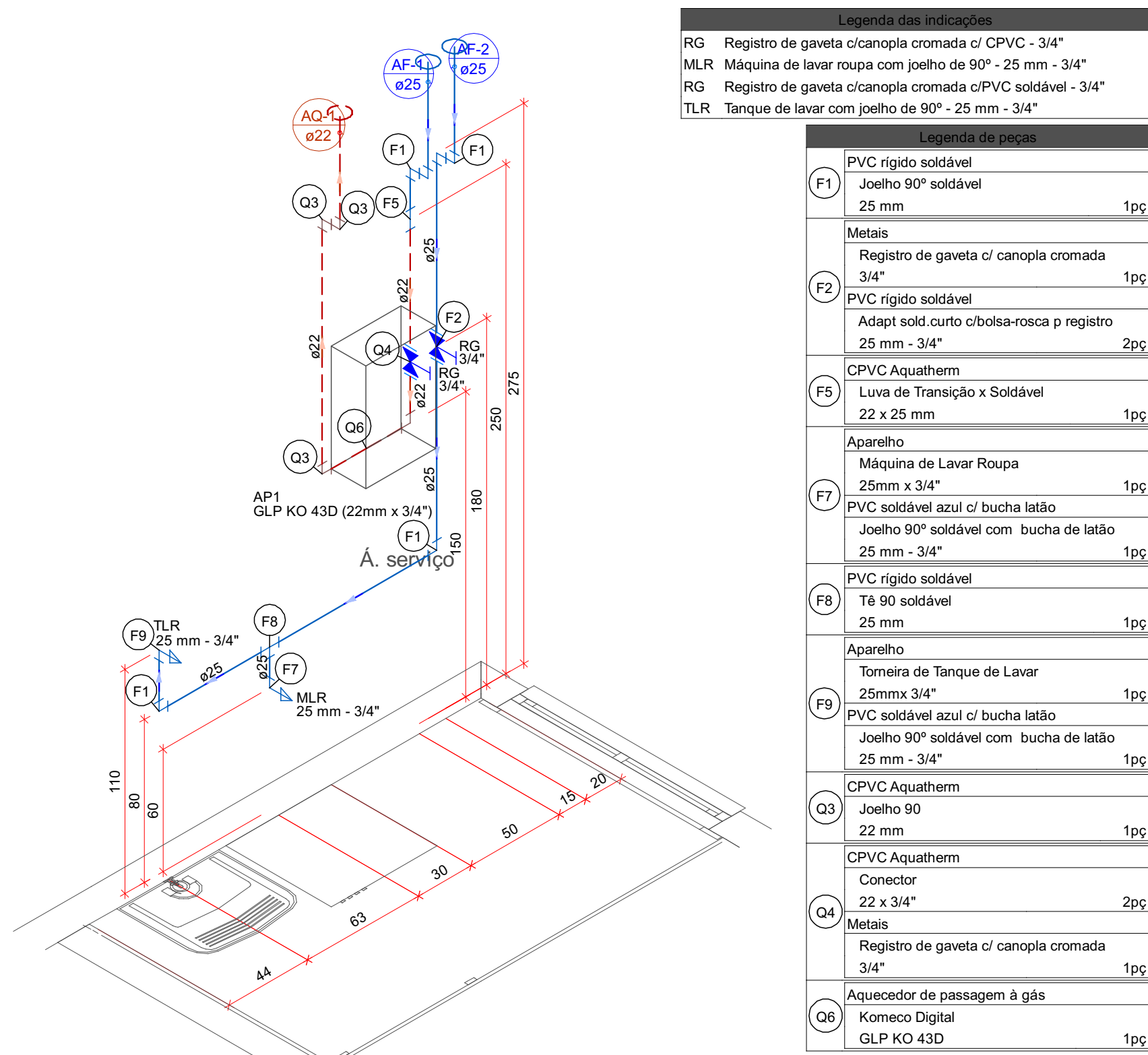
Detalhe Hidráulico-1 Escala 1:25
